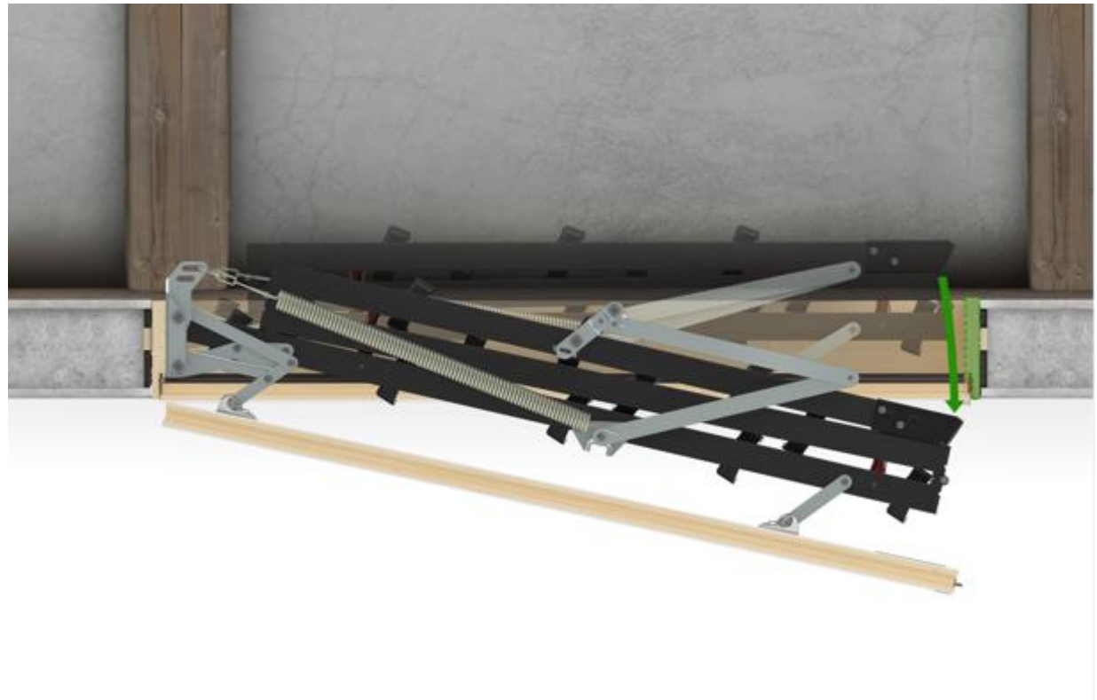
Rys. 2 Odległość zamachowa schodów ze stopkami LXS-M
