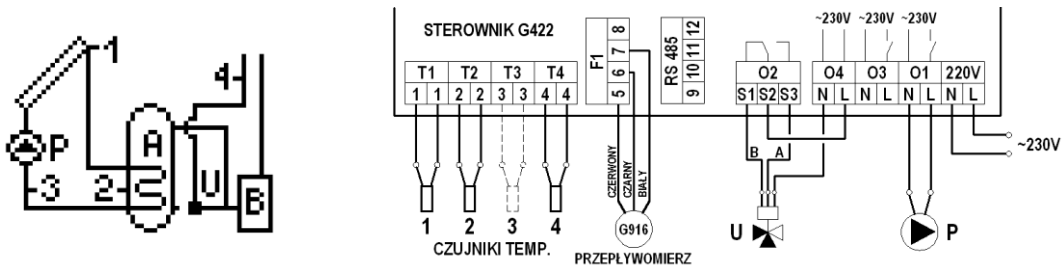
Rys. 15. Schemat ideowy oraz elektryczny instalacji układu nr 13.
