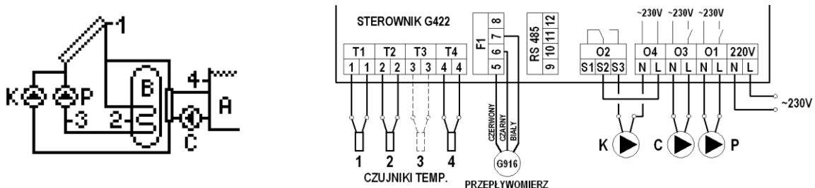
Rys. 12. Schemat ideowy oraz elektryczny instalacji nr 10.
