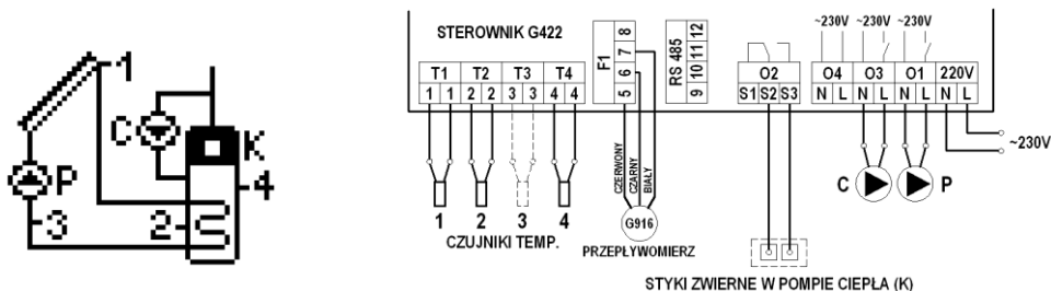
Rys. 7. Schemat ideowy oraz elektryczny instalacji nr 5.
