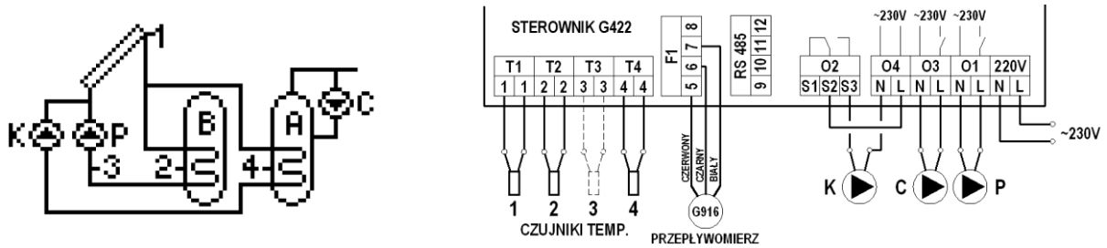
Rys. 14. Schemat ideowy oraz elektryczny instalacji układu nr 12.
