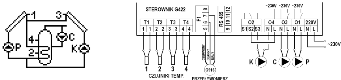
Rys. 17. Schemat ideowy oraz elektryczny instalacji układu nr 15.
