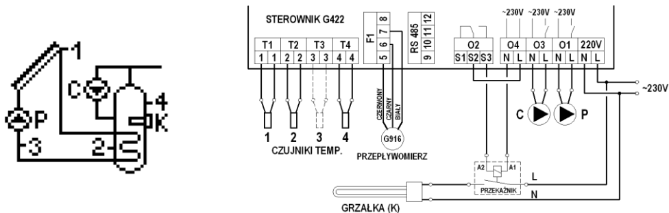
Rys. 6. Schemat ideowy oraz elektryczny instalacji nr 4.
