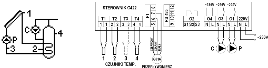
Rys. 4. Schemat ideowy oraz elektryczny instalacji nr 2.
