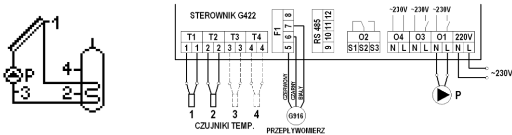
Rys. 3. Schemat ideowy oraz elektryczny instalacji nr 1.
