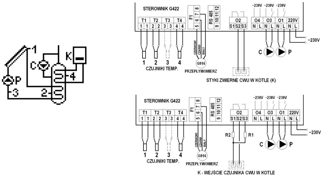
Rys. 5. Schemat ideowy oraz elektryczny instalacji nr 3.
