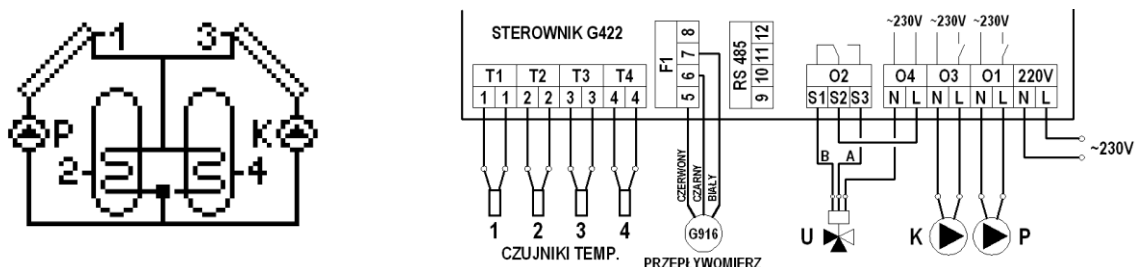
Rys. 18. Schemat ideowy oraz elektryczny instalacji układu nr 16.
