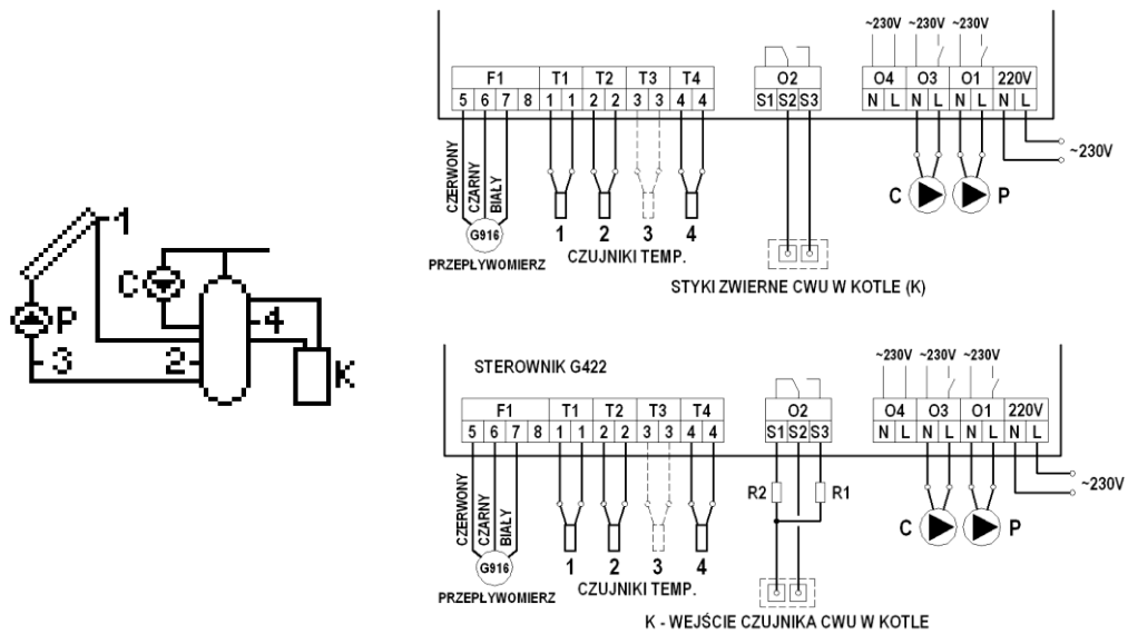
Rys. 5. Schemat ideowy oraz elektryczny instalacji nr 3.
