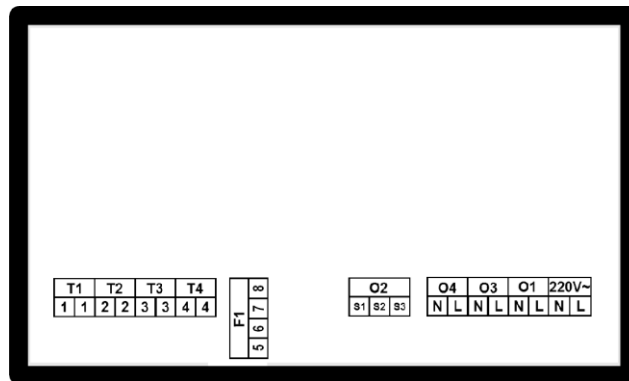
Rys. 1. Oznaczenie wejść i wyjść sterownika.
