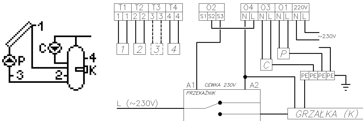
Rys. 13. Schemat ideowy oraz elektryczny instalacji nr 4.
